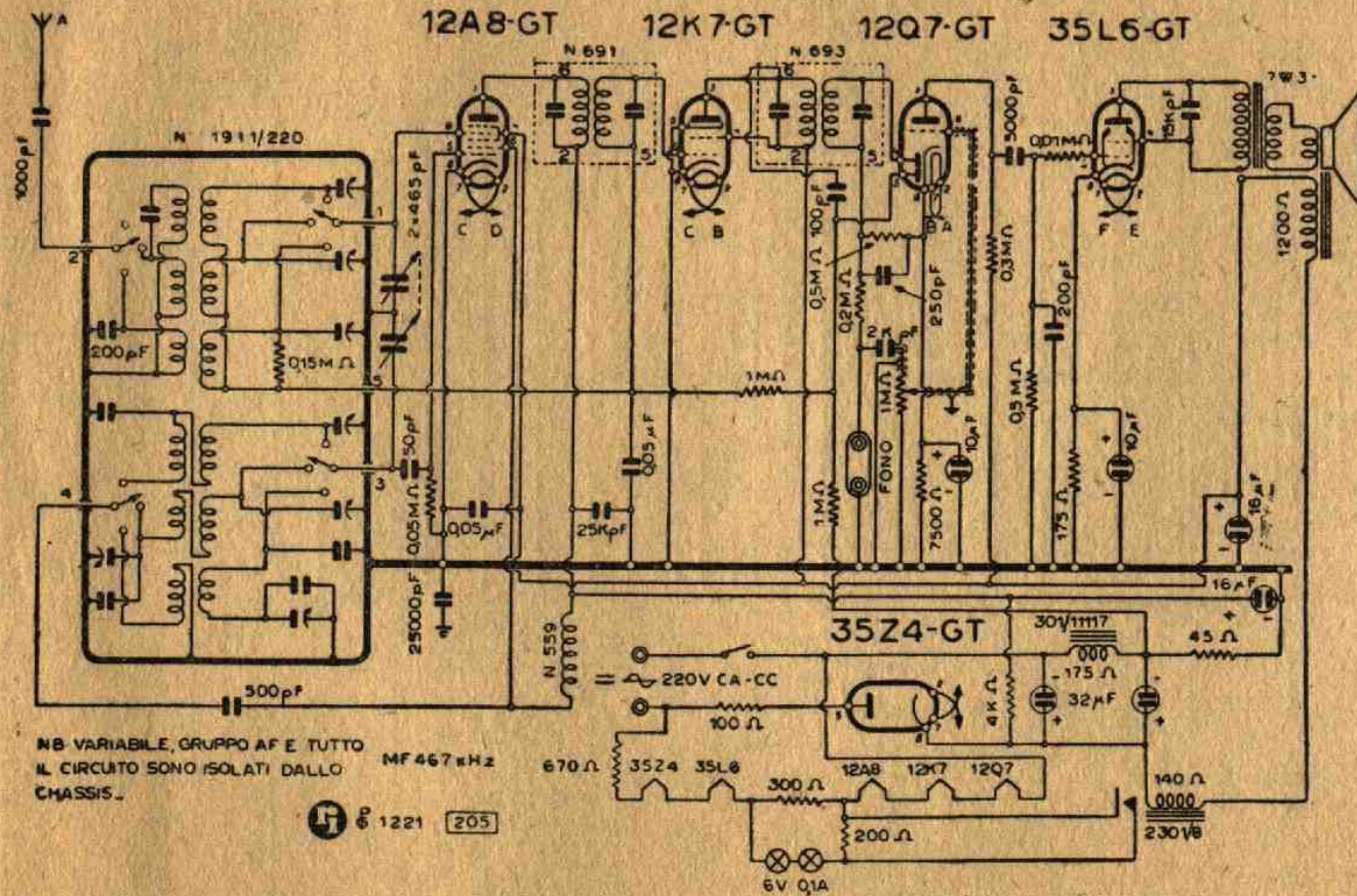
Lo schema elettrico del G-51/220 Costruttore Geloso J. s. a. - Viale Brenta, 18 - Tel. 54-183 - Milano
